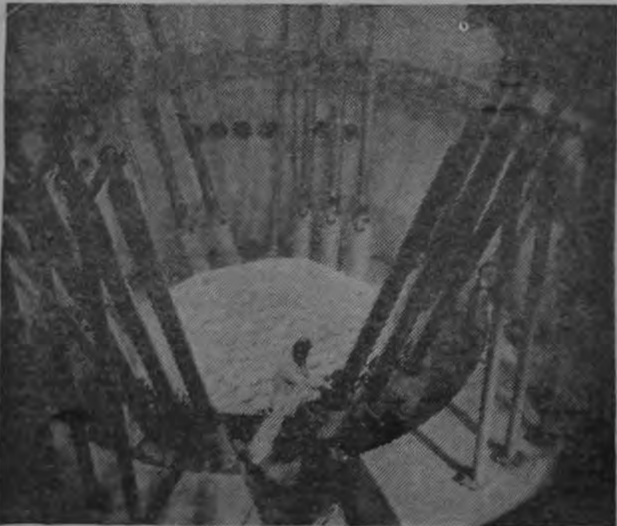
Vista de la tapa del depósito de presión del reactor. Al lado del depósito se hallan las 17 barras de control, así como los 3 tubos de entrada para inyectar ácido bórico. Las barras de control inclinadas sirven para regular y desconectar rápidamente el reactor.
